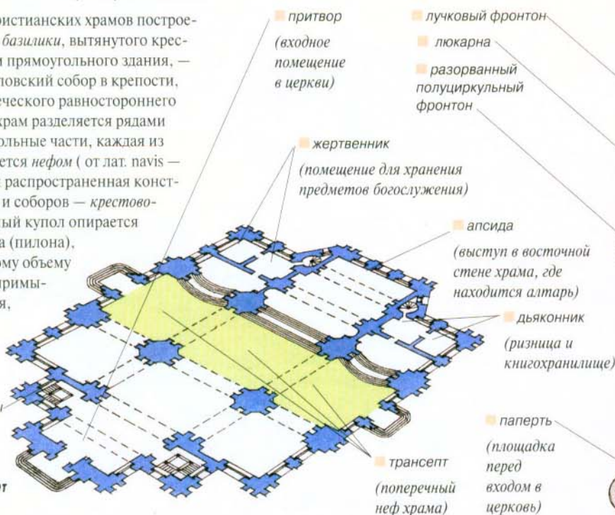
План Петропавловского собора — трехнефной базилики
