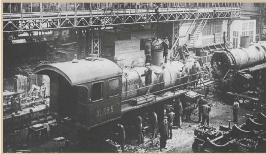
Паровозремонтная мастерская Путиловского завода. Фотография
