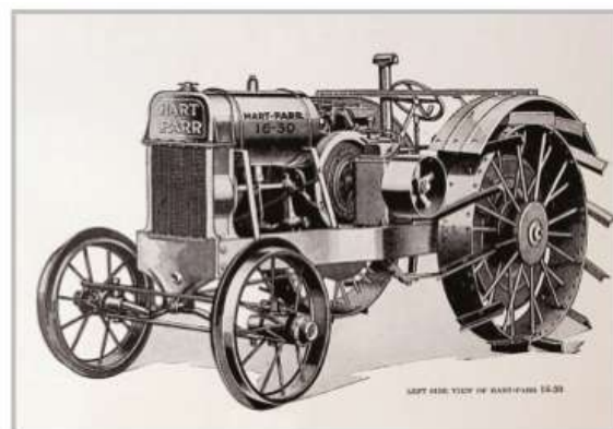
Трактор «Харт — Парр 1630». Рисунок 1928 г.
