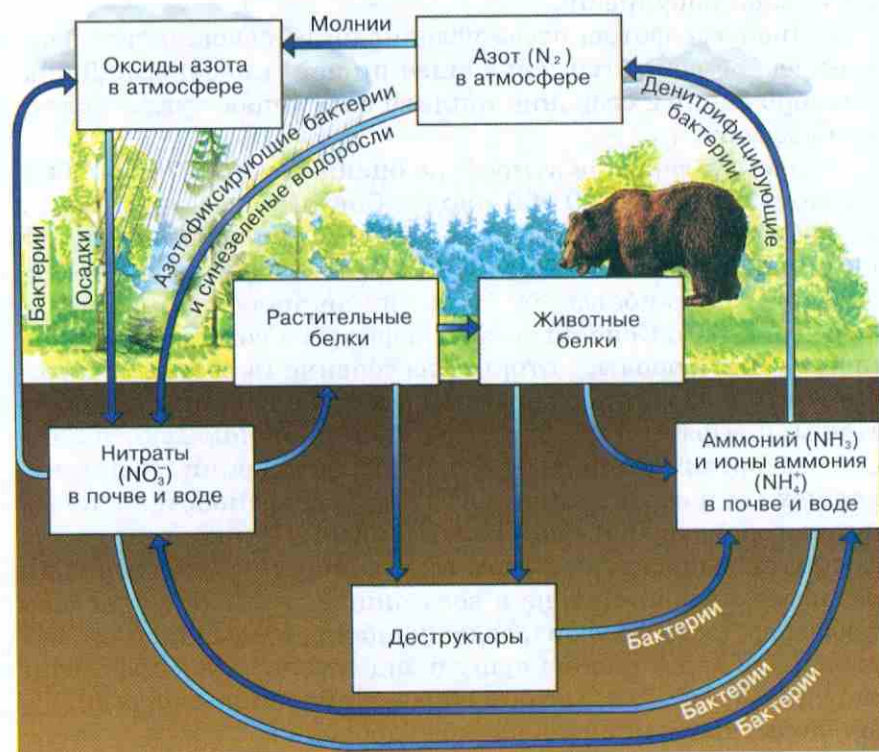
Рис. 68. Биогеохимический цикл азота
