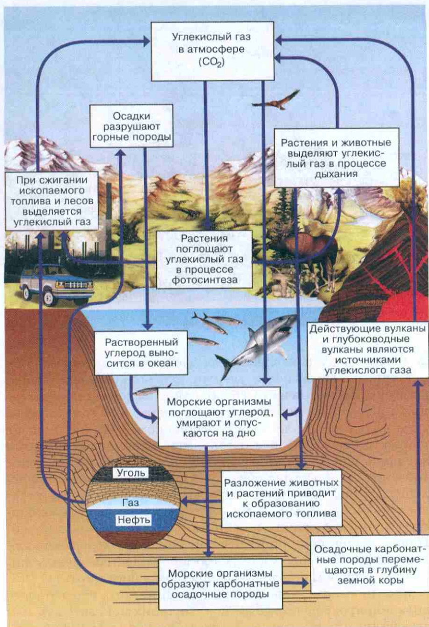
Рис. 69. Биогеохимический цикл углерода
