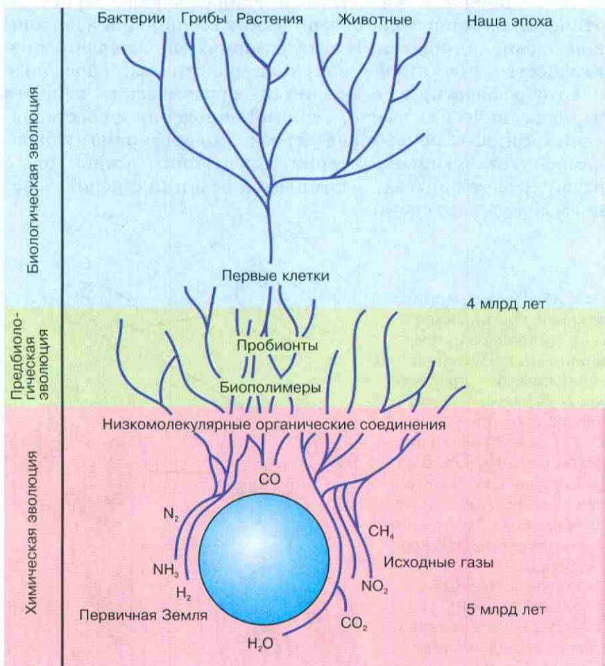
Рис. 87. Основные этапы развития жизни
