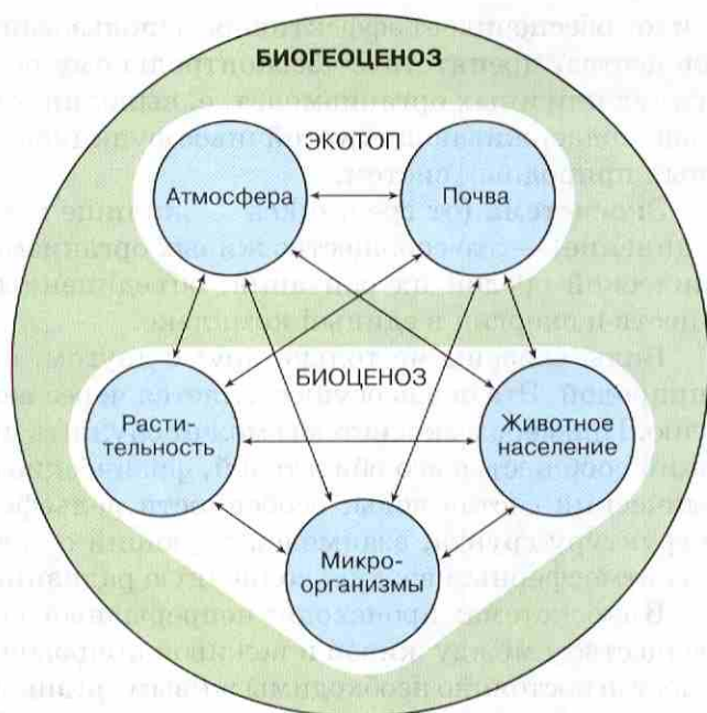
Рис. 59. Схема биогееоценозов
