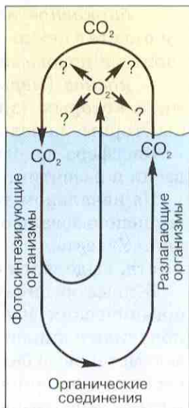
Рис. 109. Схема круговорота углерода с появлением организмов с современным механизмом фотосинтеза
