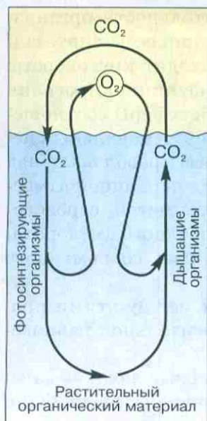
Рис. 110. Схема круговорота с появлением у организмов процесса дыхания
