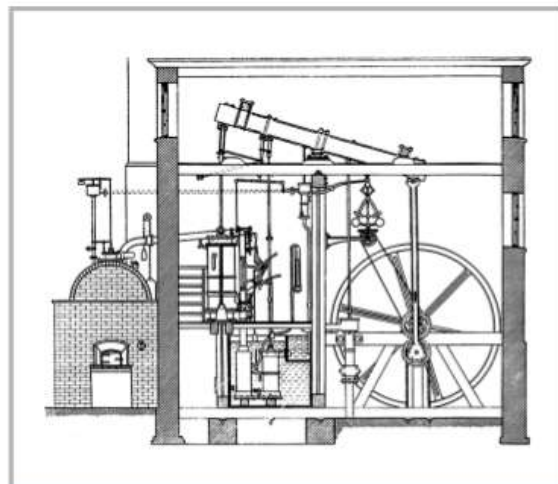
Чертеж двигателя паровой машины Дж. Уатта. XVIII в.
