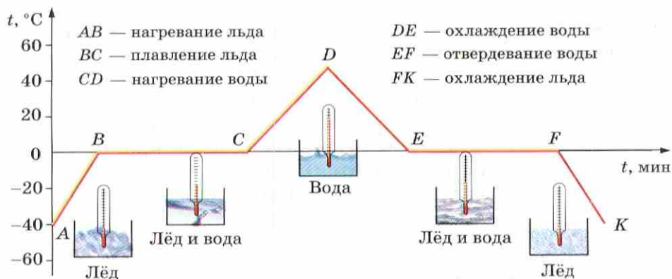
Рис. 18. График зависимости температуры льда от времени нагревания
