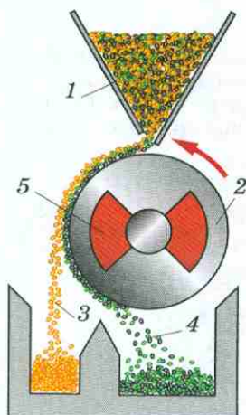
Рис. 104. Магнитный сепаратор
