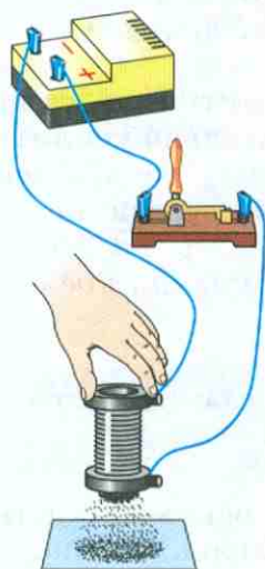
Рис. 97. Притяжение железных опилок катушкой с током
