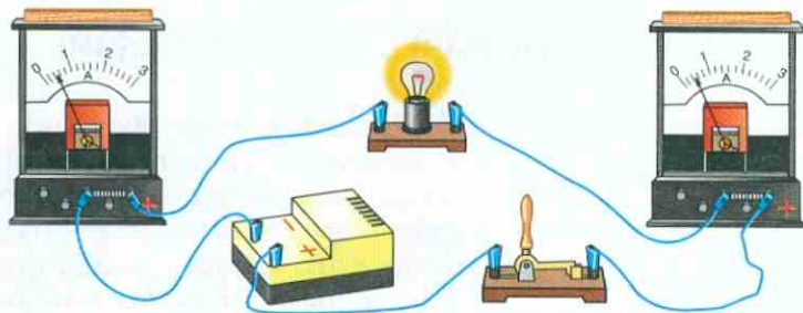
Рис. 62. Измерение силы тока на разных участках цепи
