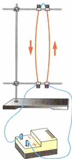
Рис. 60. Взаимодействие проводников с током
