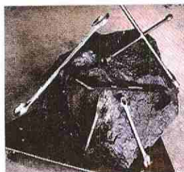
Рис. 110. Притяжение металлических тел естественным магнитом
