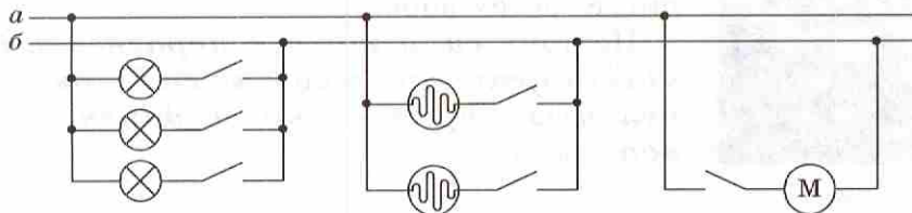
Рис. 81. Параллельное включение в цепь различных потребителей
