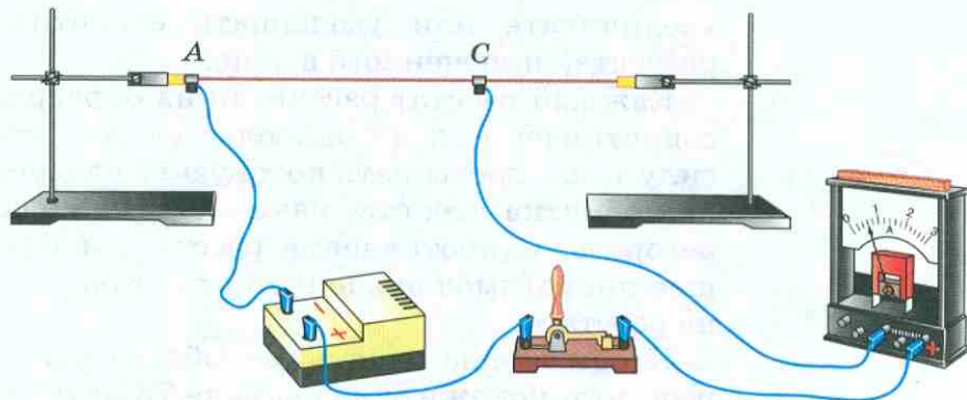
Рис. 75. Изменение длины проводника, включённого в цепь
