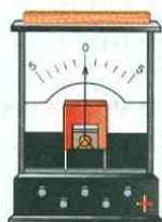
Рис. 57. Рамка с током неподвижна
