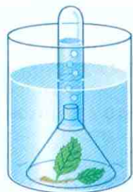
Рис. 17. Превращение солнечной энергии в химическую энергию
