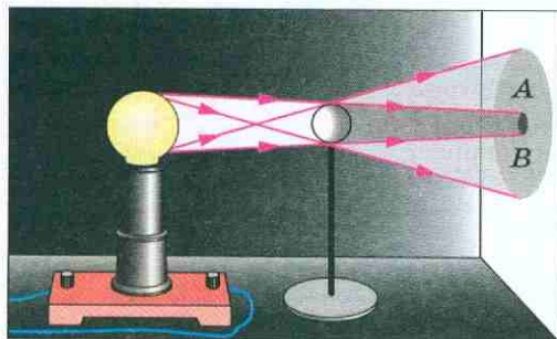
Рис. 124. Получение полутени
