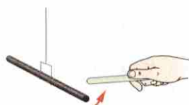
Рис. 32. Притяжение наэлектризованных палочек
