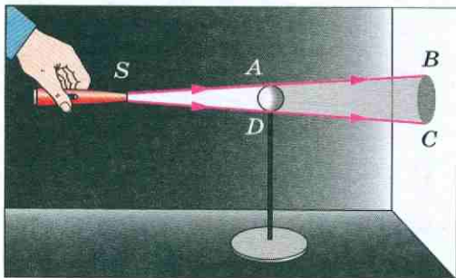
Рис. 123. Получение тени
