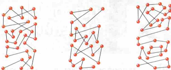
Рис. 1. Траектория движения микрочастиц краски, растворённой в воде
