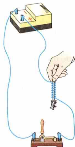
Рис. 56. Магнитное действие тока
