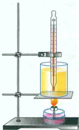
Рис. 15. Нагревание разных веществ равной массы
