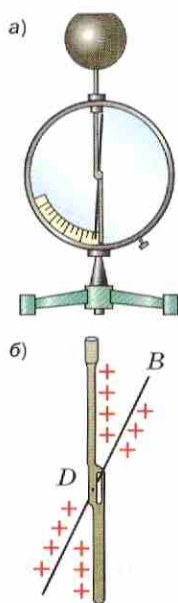
Рис. 35. Электрометр: а — внешний вид; б — механизм зарядки
