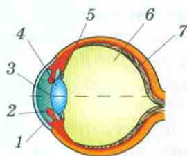
Рис. 163. Глаз человека
