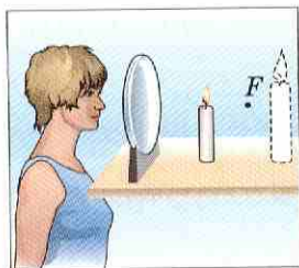
Рис. 157. Прямое изображение свечи
