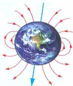
Рис. 116. Магнитные линии магнитного поля Земли
