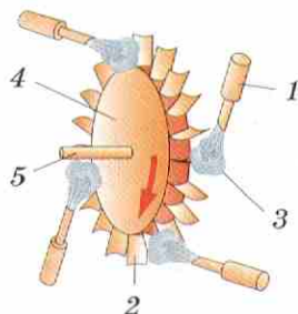
Рис. 28. Схема паровой турбины
