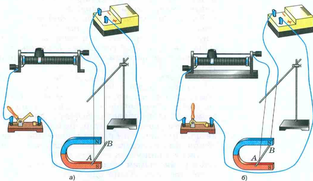
Рис. 117. Действие магнитного поля на проводник с током
