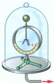
Рис. 36. Заряженный электроскоп под колоколом воздушного насоса
