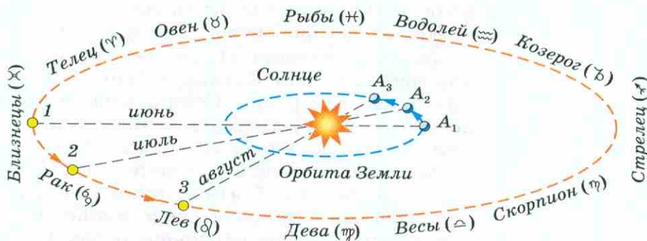
Рис. 131. Движение Земли вокруг Солнца и кажущееся годичное движение Солнца
