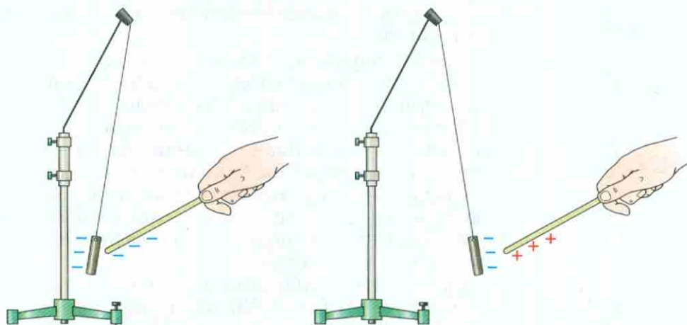
Рис. 33. Электризация гильзы
