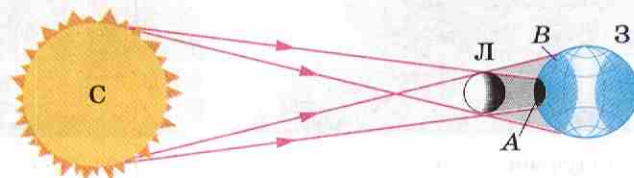
Рис. 126. Солнечное затмение
