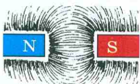
Рис. 113. Магнитные линии магнитного поля, созданного двумя магнитами
