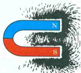
Рис. 112. Картина магнитного поля полосового и дугообразного магнитов
