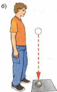
Рис. 2. Превращение механической энергии свинцового шара
