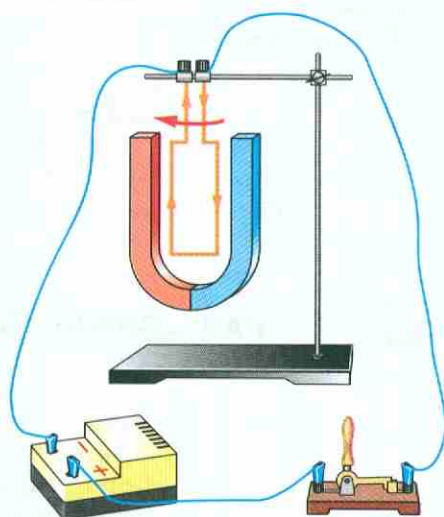
Рис. 58. Рамка с током между полюсами магнита поворачивается
