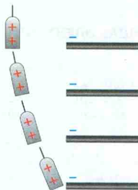
Рис. 37. Зависимость действия электрического поля от расстояния до заряда
