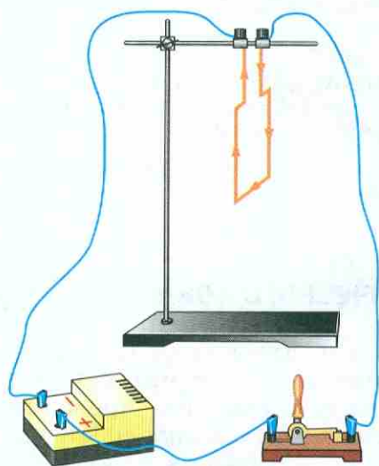
Рис. 57. Рамка с током неподвижна
