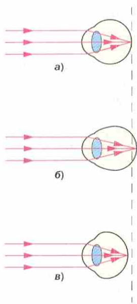
Рис. 165. Недостатки зрения
