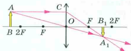
Рис. 158. Изображение, даваемое линзой, когда расстояние от источника света больше двойного фокуса
