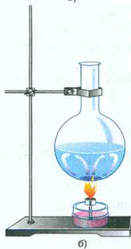
Рис. 9. Конвекция: а — в воздухе; б — в жидкостях
