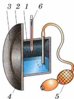
Рис. 23. Внешний вид и устройство конденсационного гигрометра
