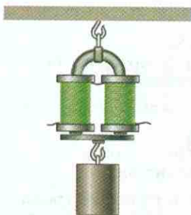
Рис. 102. Дугообразный электромагнит
