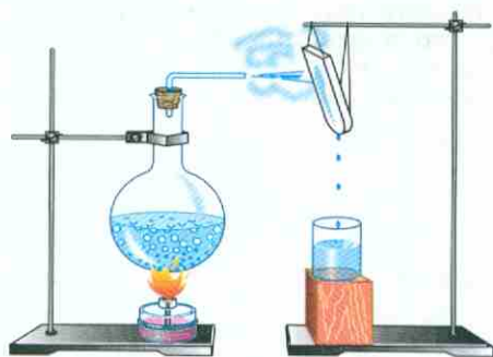
Рис. 25. Конденсация пара
