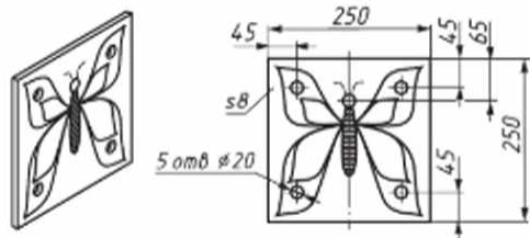
Рис. 2.1. Технологическая карта на изготовление подставки под горячее
