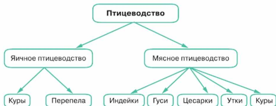
Рис. 14.2. Направления птицеводства
