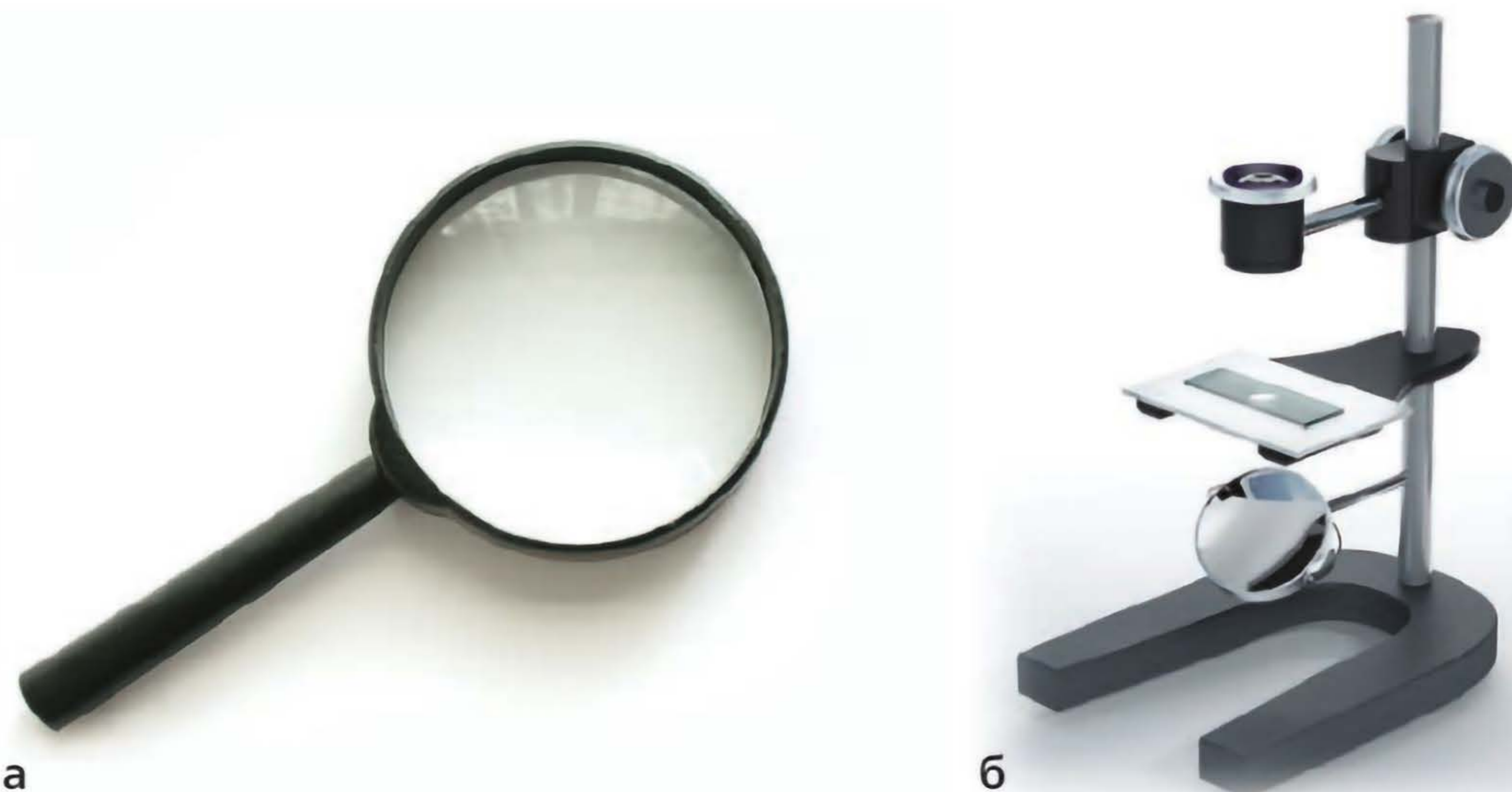
Рис. 43. Лупы ручная (а) и штативная (б)
