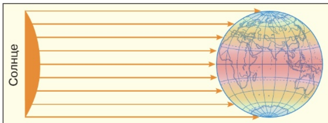
Схема нагрева поверхности Земли солнечными лучами
