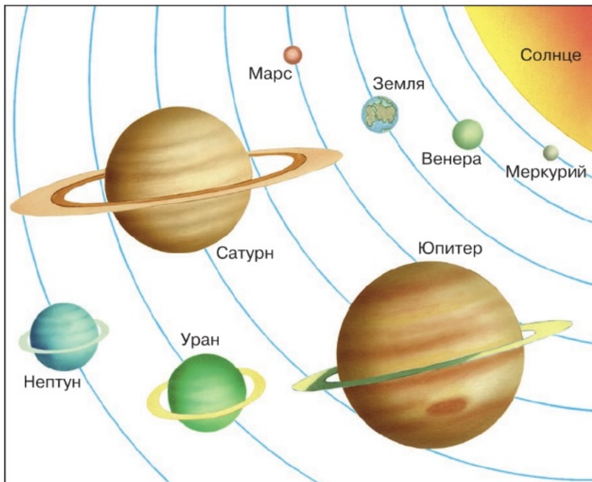
Солнечная система
