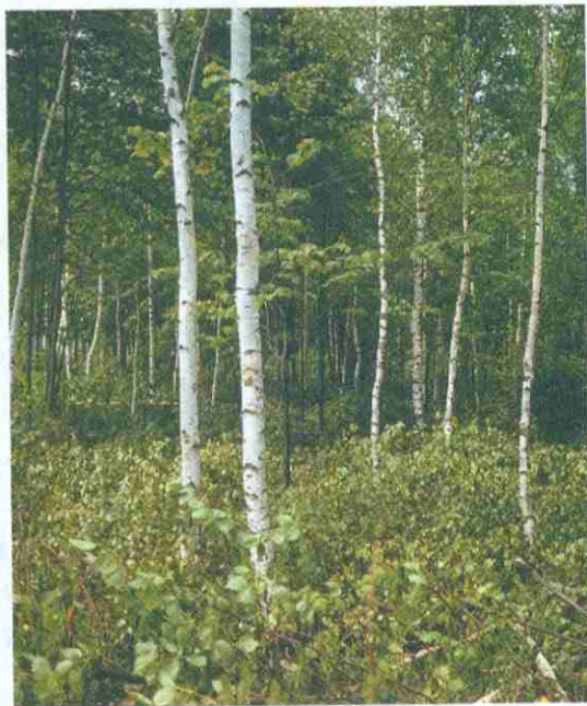
Рис. 103. Экосистема листопадного леса
