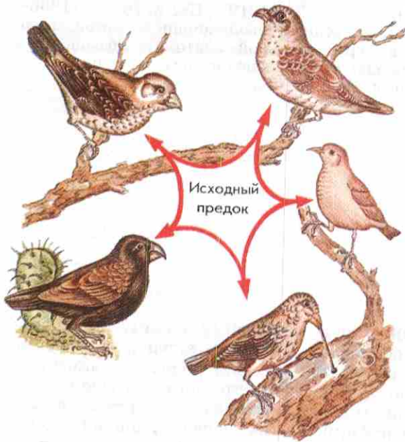
Рис. 65. Разнообразие вьюрков на Галапагосских островах
