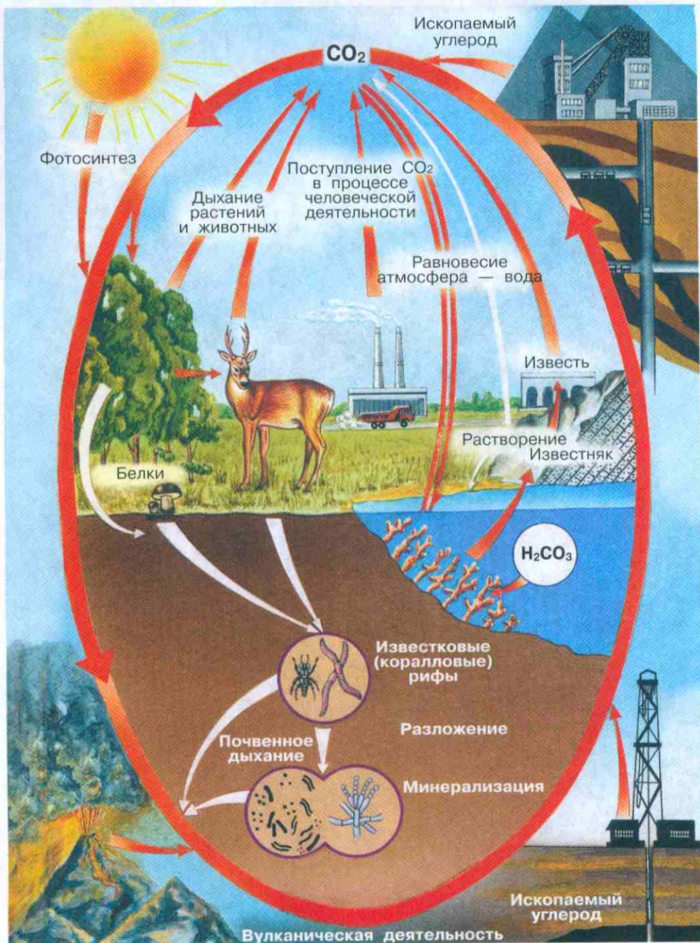
Рис. 107. Круговорот углерода
