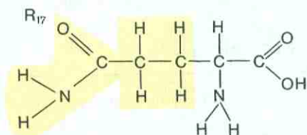
Глутамин (гln)
