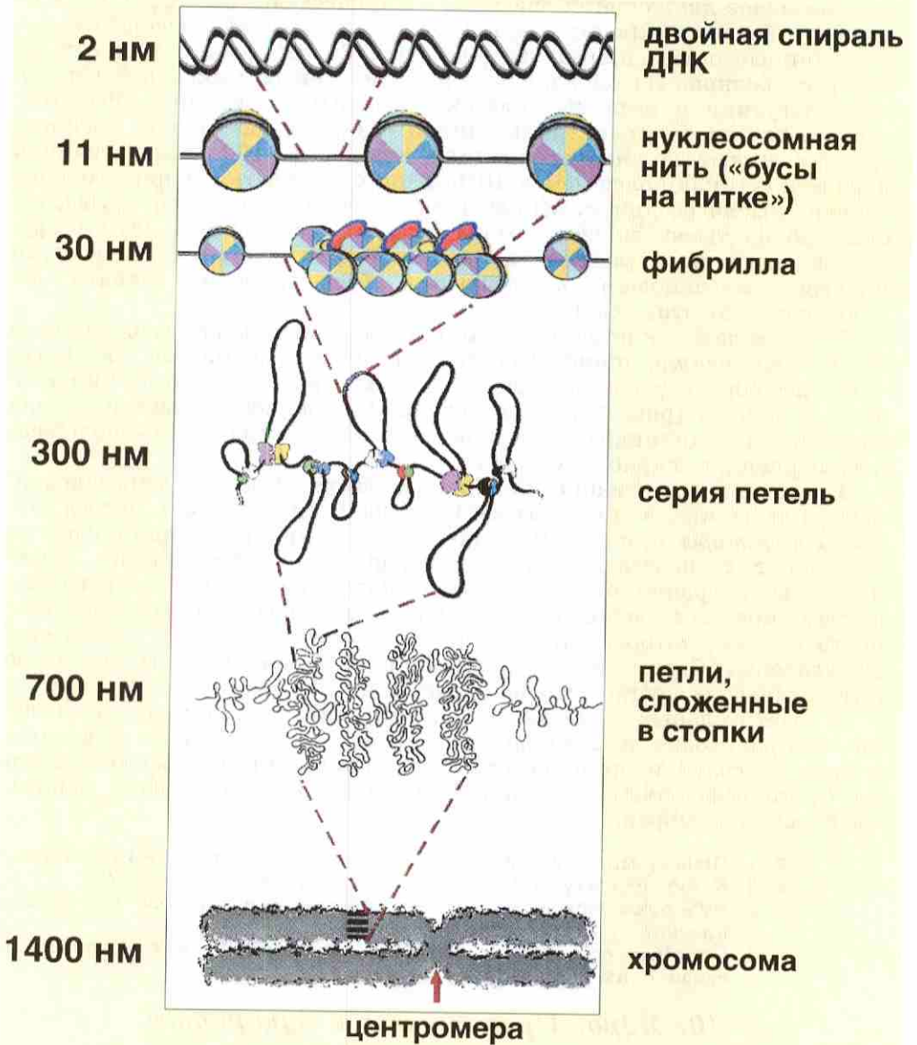
Рис. 17. Схема упаковки ДНК в хромосоме
