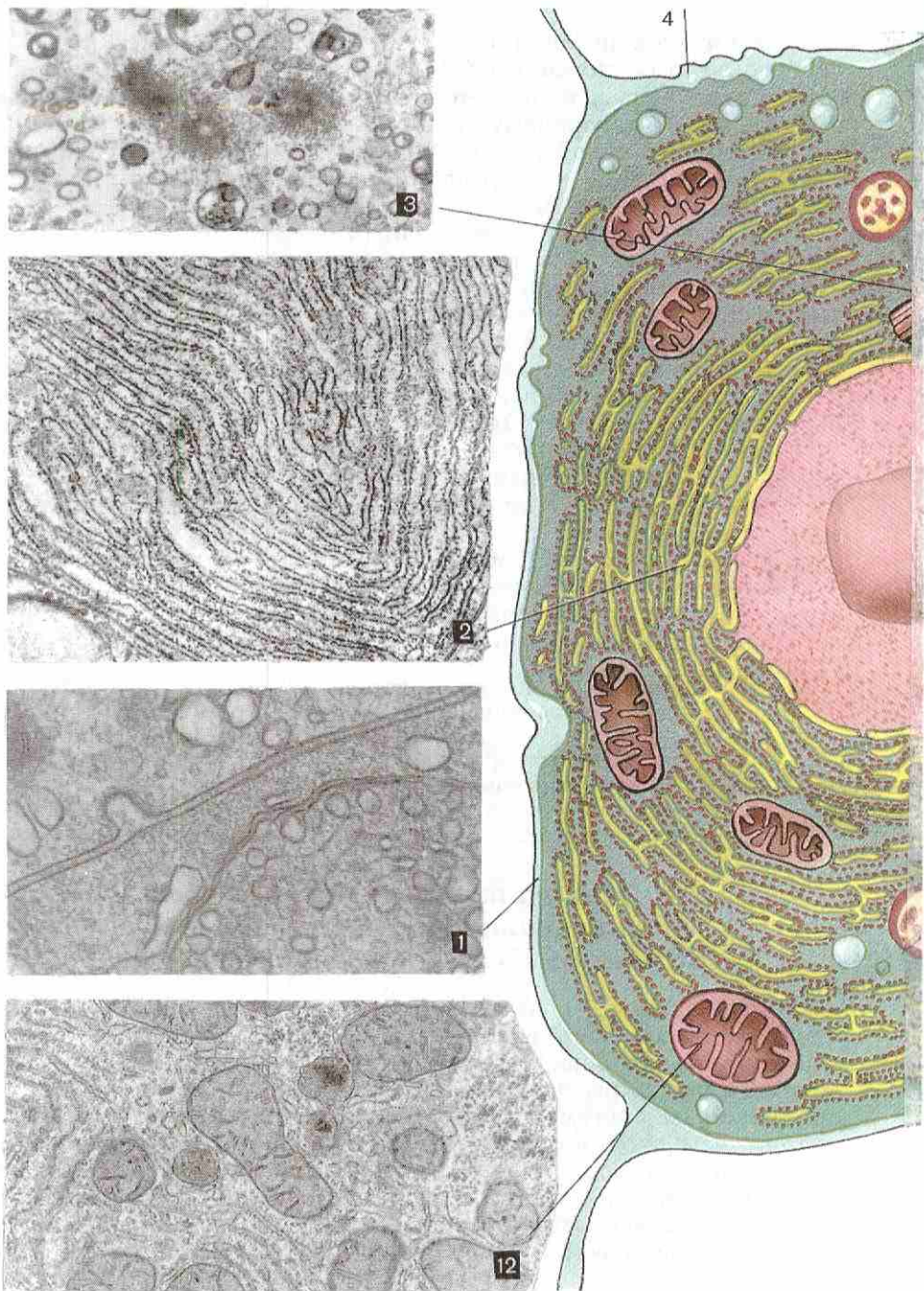
Рис. 11. Клетка под электронным микроскопом. 1 — плазматическая мембрана; 2 — эндоплазматическая сеть; 3 — центриоль; 4 — межклеточное пространство; 5 — пиноцитозный канал;
