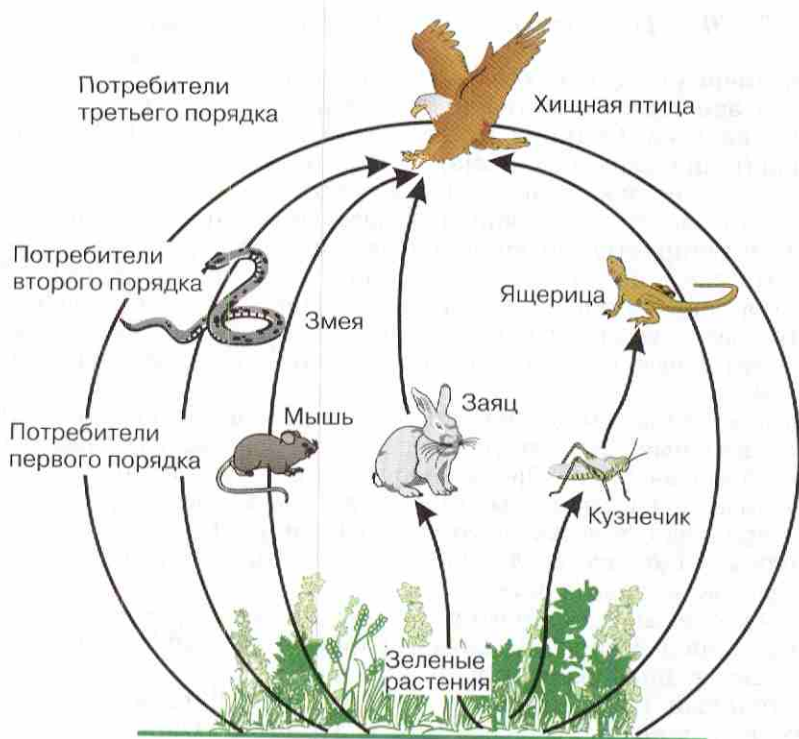
Рис. 104. Пищевые цепи в наземных экосистемах
