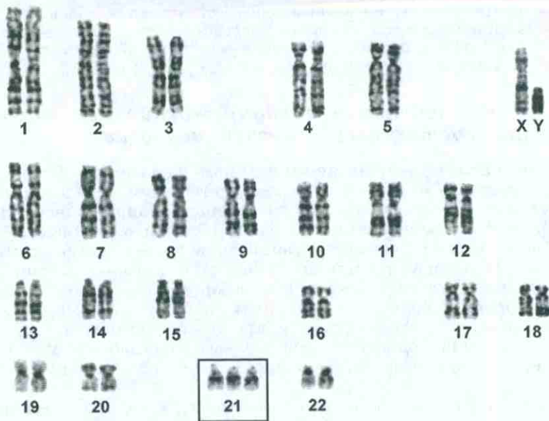
Рис. 49. Хромосомный набор мужчины с болезнью Дауна
