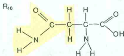
Аспарагин (асн)
