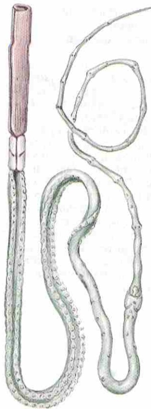
Рис. 83. Погонофора
