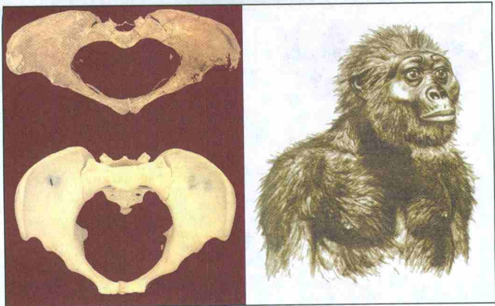
Рис. 93. Австралопитек афарский.
