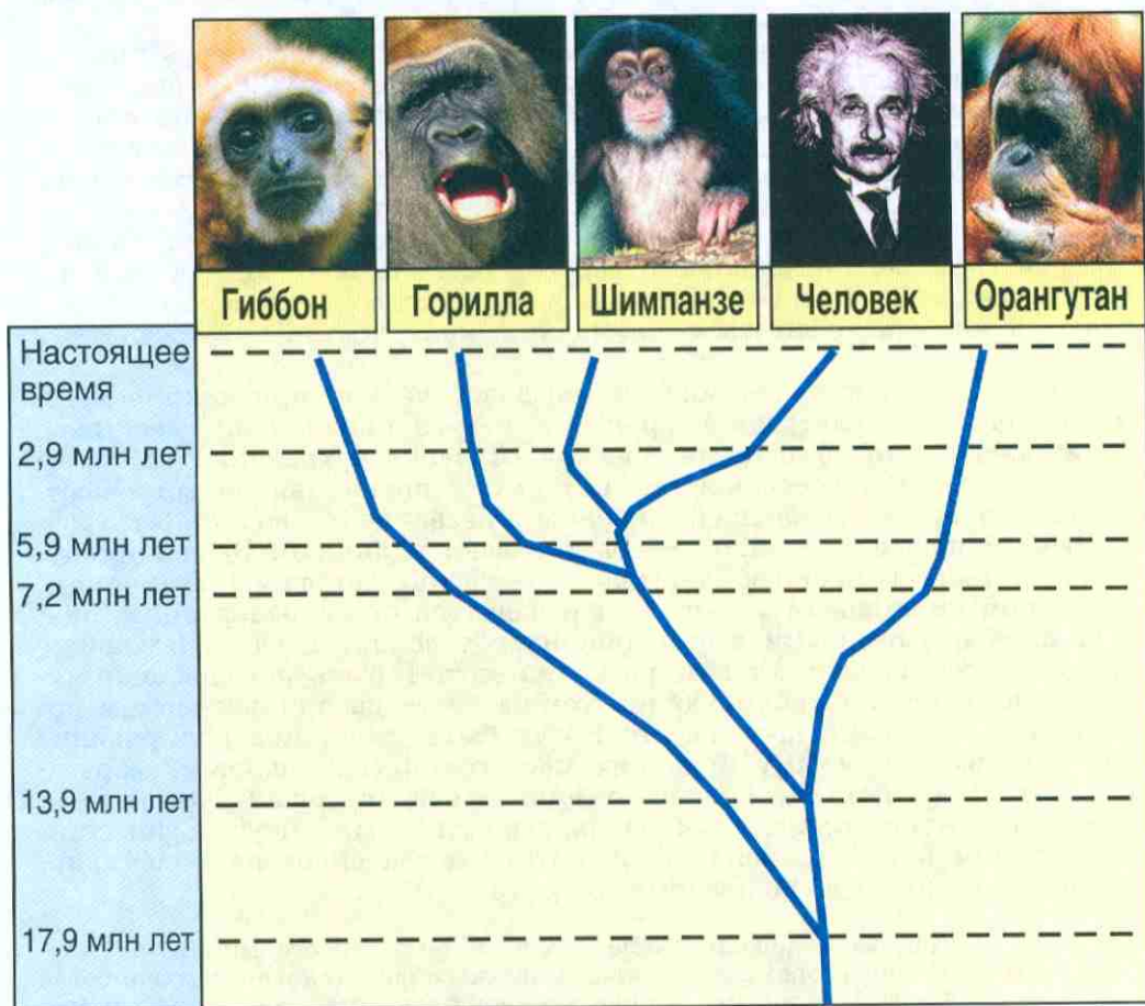
Рис. 92. Филогенетическое древо гоминоидов, основанное на структуре глобиновых генов
