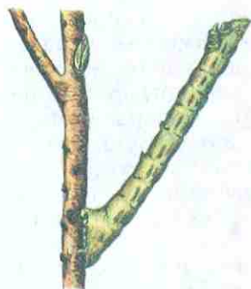
Рис. 62. Покровительственная форма гусеницы (напоминающая сучок) защищает ее от врагов
