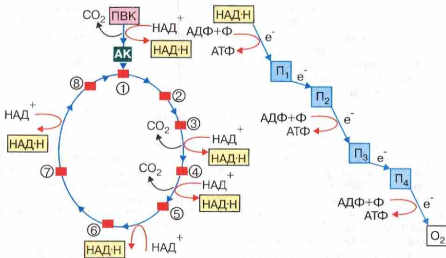
Рис. 20. Биологическое окисление с участием кислорода.
