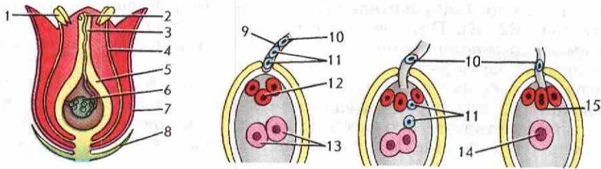
Рис. 33. Двойное оплодотворение у цветковых растений.
