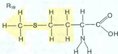
Метионин (мет) *
