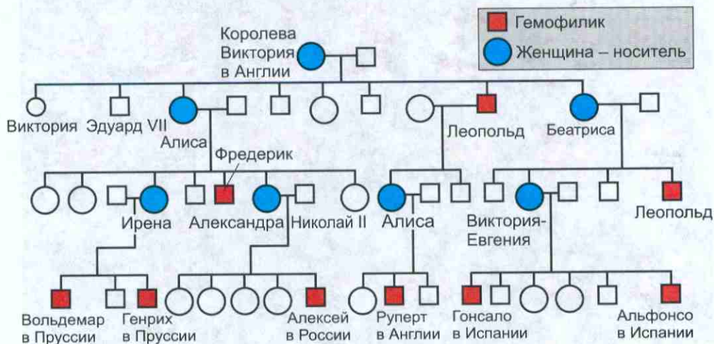
Рис. 46. Наследование гемофилии
