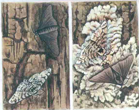
Рис. 58. Индустриальный меланизм у бабочек
