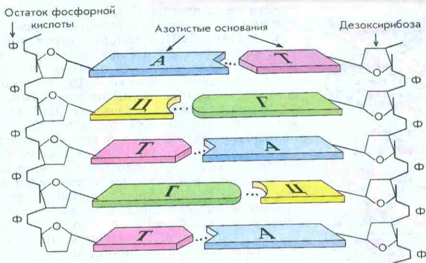
Рис. 7. Схема строения ДНК. Многоточием обозначены водородные связи
