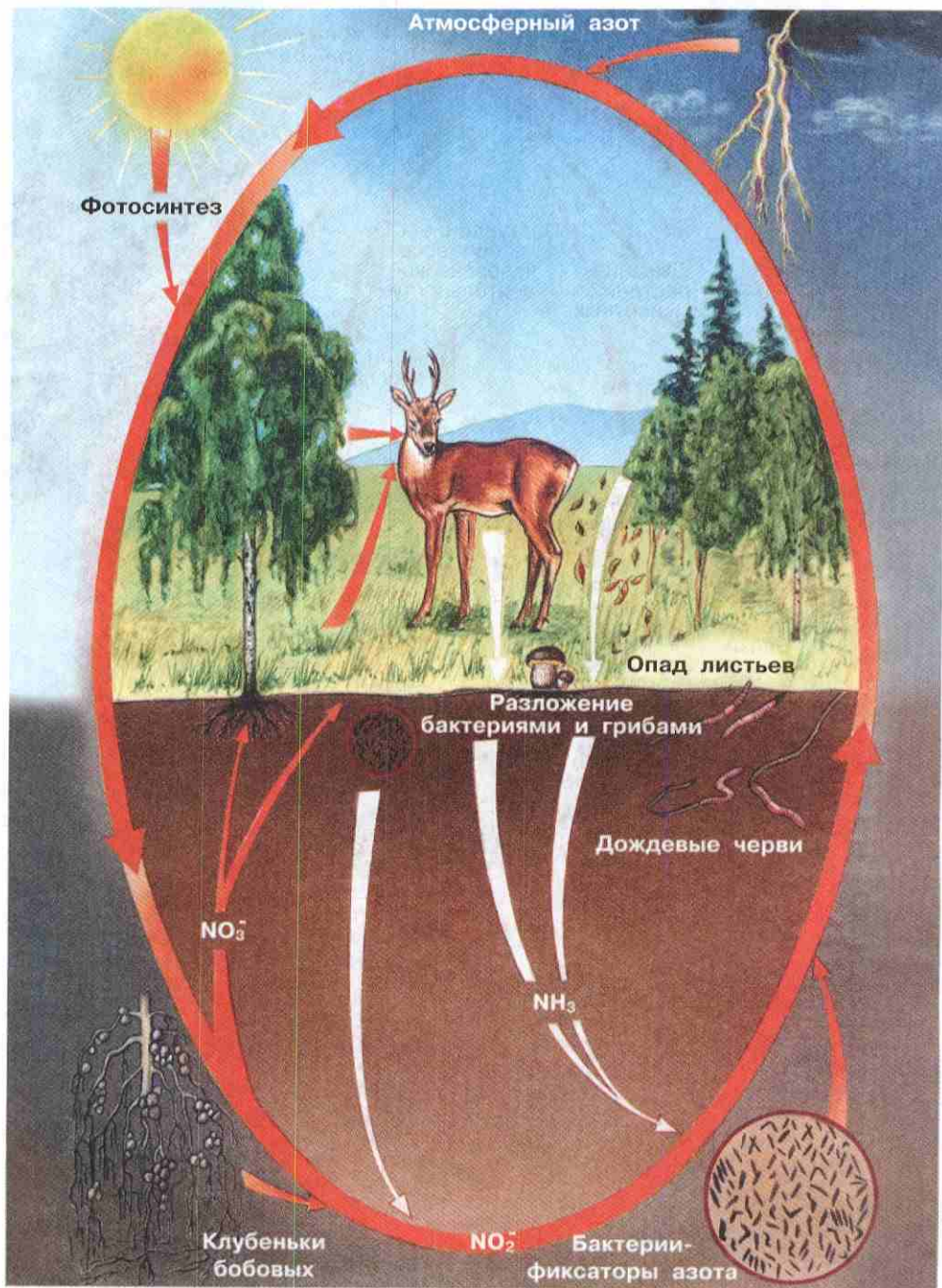
Рис. 108. Круговорот азота
