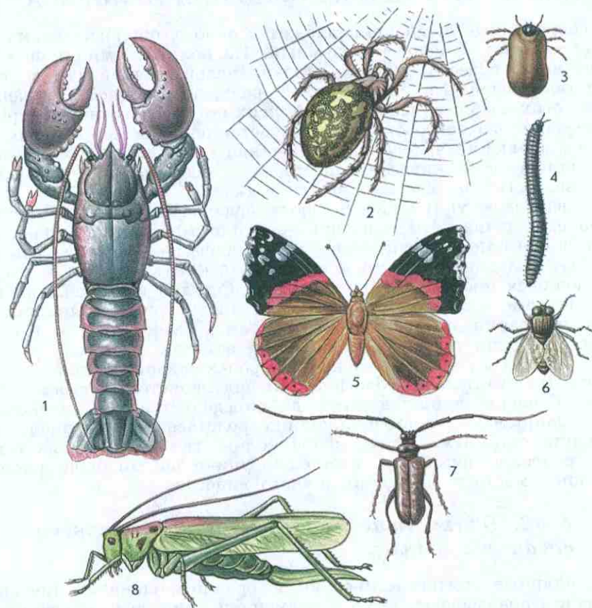
Рис. 89. Представители членистоногих.
