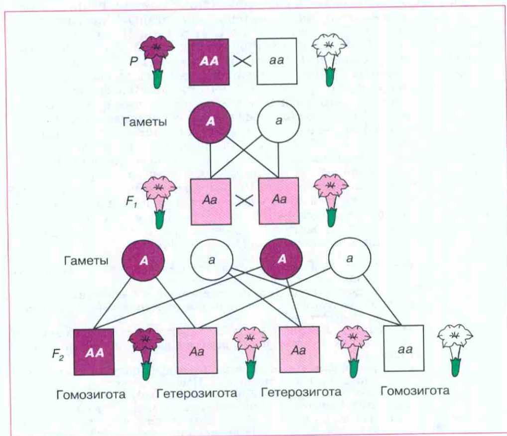
Рис. 36. Промежуточное наследование у ночной красавицы
