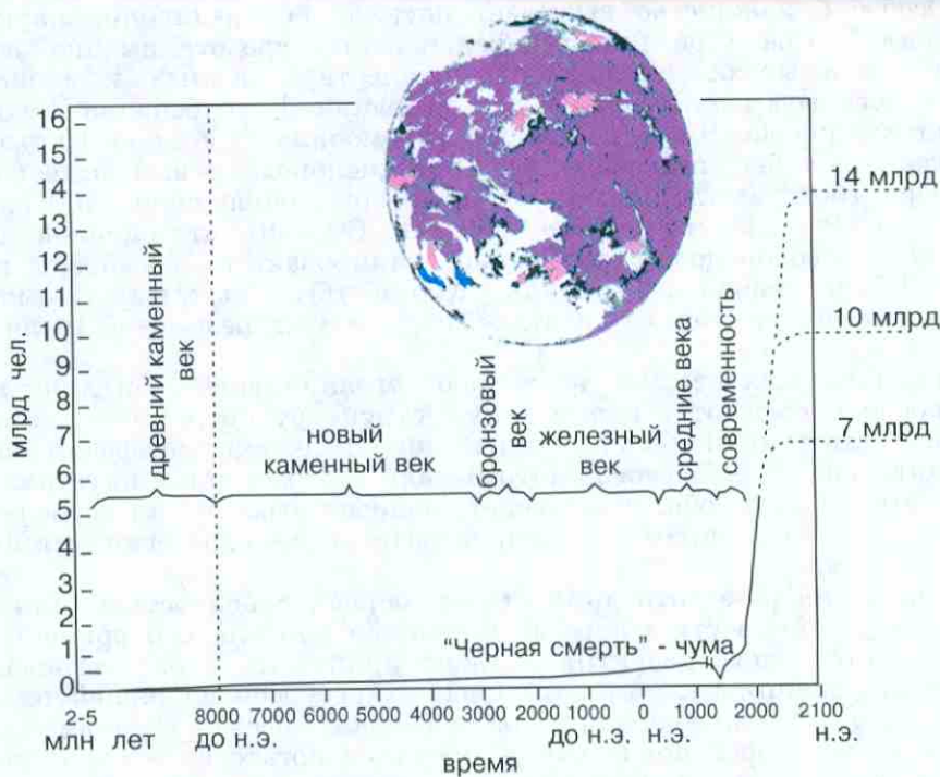
Рис. 110. График экспоненциального роста численности населения в прошлом и прогнозе на 2100 г.
