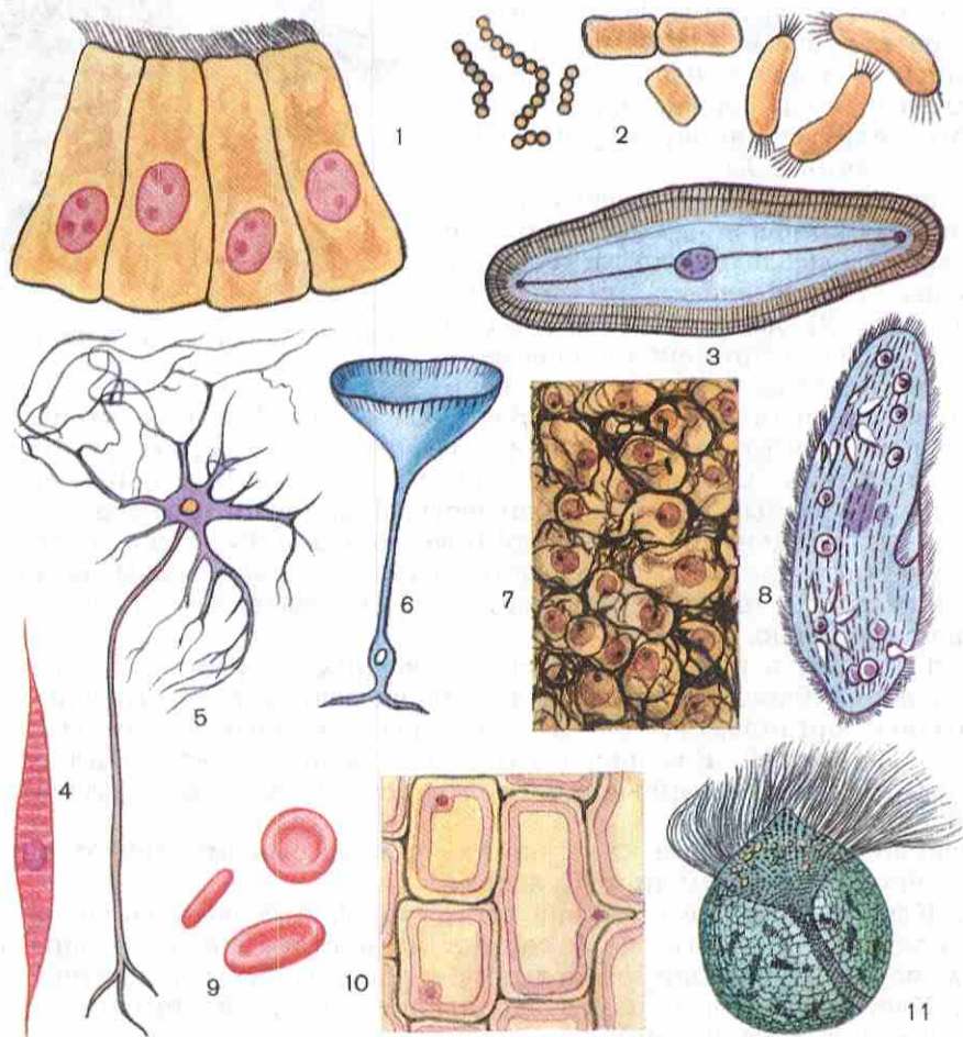
Рис. 10. Различные формы клеток в связи с выполняемыми функциями. 1 — клетки эпителия кишечника; 2 — бактерии (кокки, кишечная палочка, спириллы со жгутиками на концах тела); 3 — диатомовая водоросль; 4 — мышечная клетка; 5 — нервная клетка; 6 — одноклеточная водоросль ацетабулярия; 7 — клетки печени; 8 — инфузория; 9 — эритроциты человека; 10 — клетки эпидермиса лука; 11 — жгутиконосец
