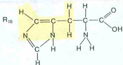
Гистидин (гис) *
