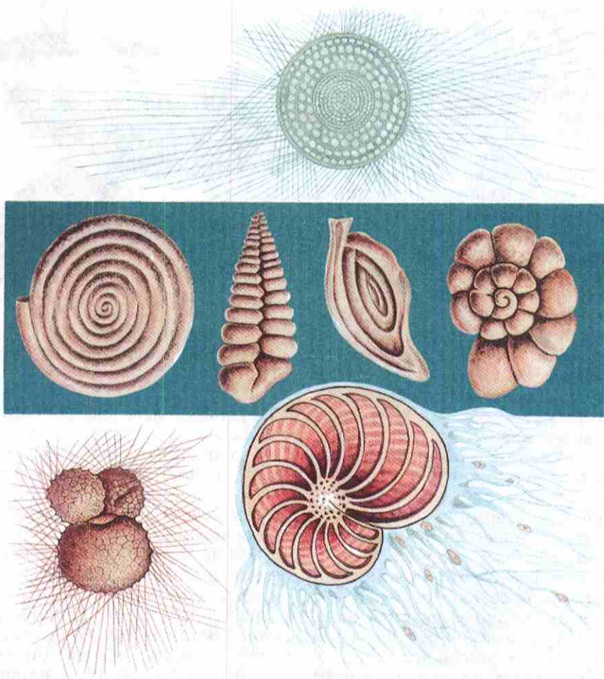
Рис. 79. Фораминиферы.
