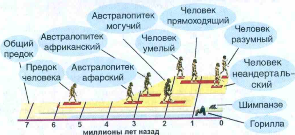
Рис. 100. Общая схема эволюции гоминоидов
