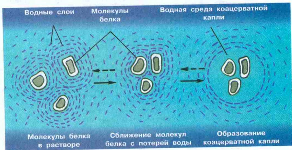
Рис. 70. Образование коацерватной капли
