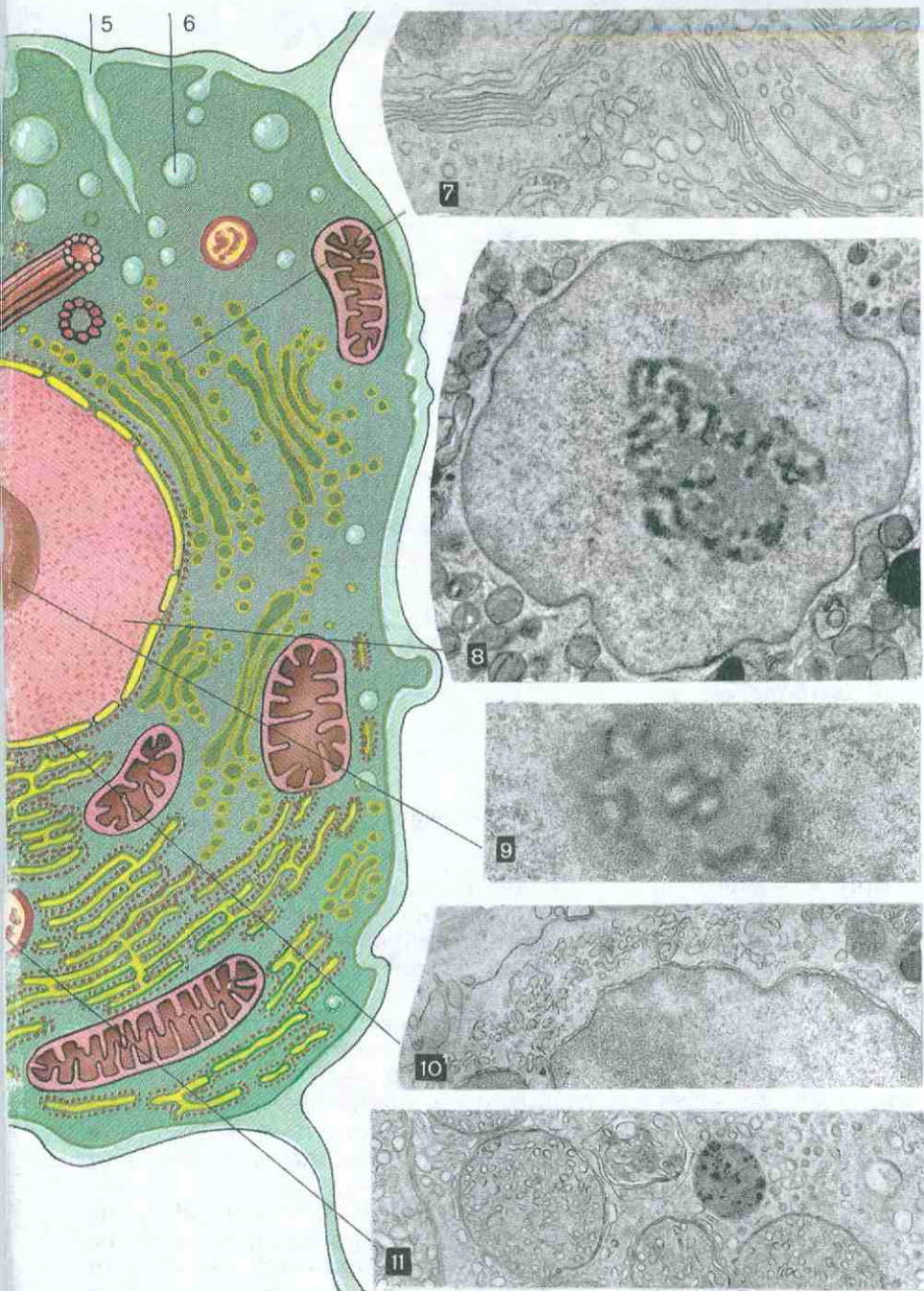
6 — пиноцитозный пузырек; 7 — комплекс Гольджи; 8 — ядро; 9 — ядрышко; 10 — ядерная оболочка; 11 — лизосома; 12 — митохондрия
