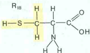
Цистеин (цис)
