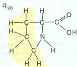
Пролин (про)
