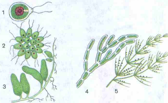
Рис. 86. Настоящие водоросли.
