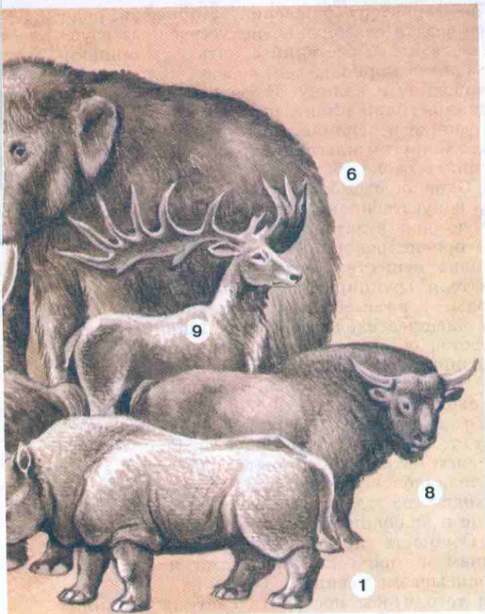
Рис. 82. Млекопитающие плейстоцена.
